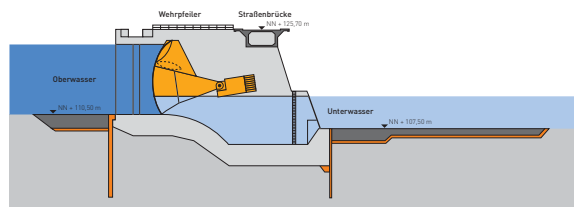
Längsschnitt Wehr.
