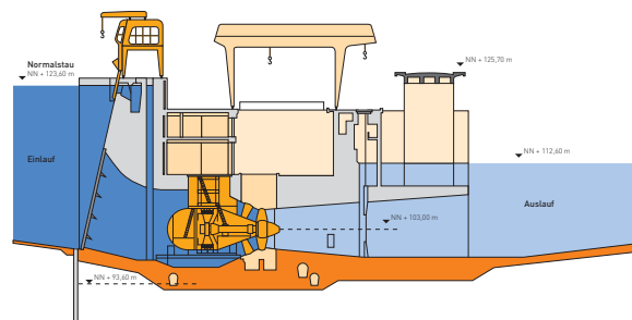
Längsschnitt Kraftwerk.
